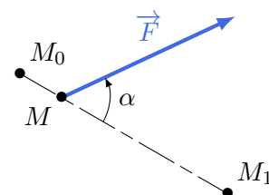
FIGURE 2 – Travail élémentaire de \vec{F}
