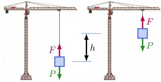
FIGURE 1 – Énergie, travail, puissance
